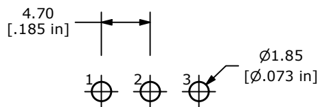
P.C MOUNT
