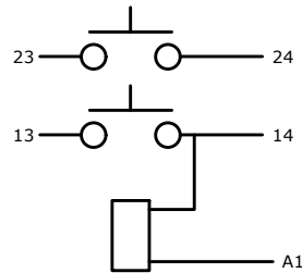
CIRCUIT: DPST
