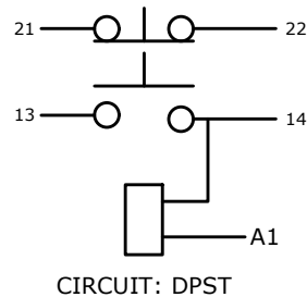
CIRCUIT: DPST
