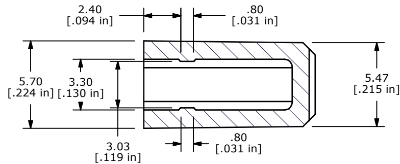
SECTION A-A SCALE 4 : 1
