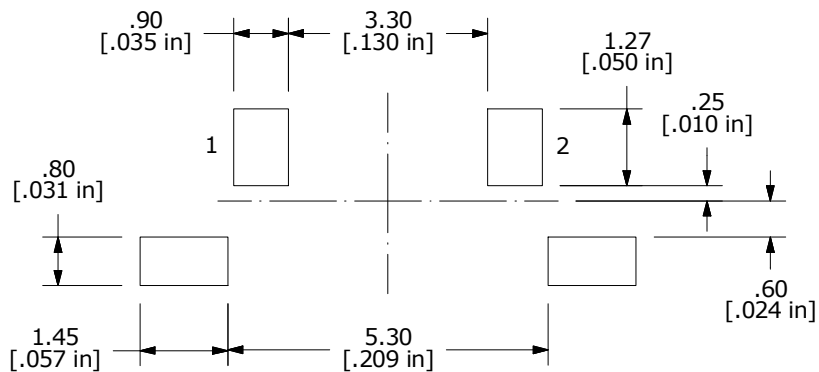
P.C.B. LAYOUT
