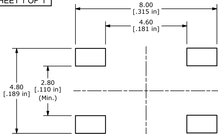
P.C. LAYOUT
